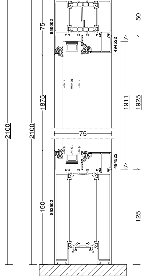
B-B
